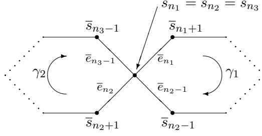
FIGURE 4. Illustration du lemme 4.6, dans \Gamma_0 \backslash X
