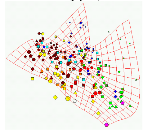
вид карты в пространстве главных компонент
